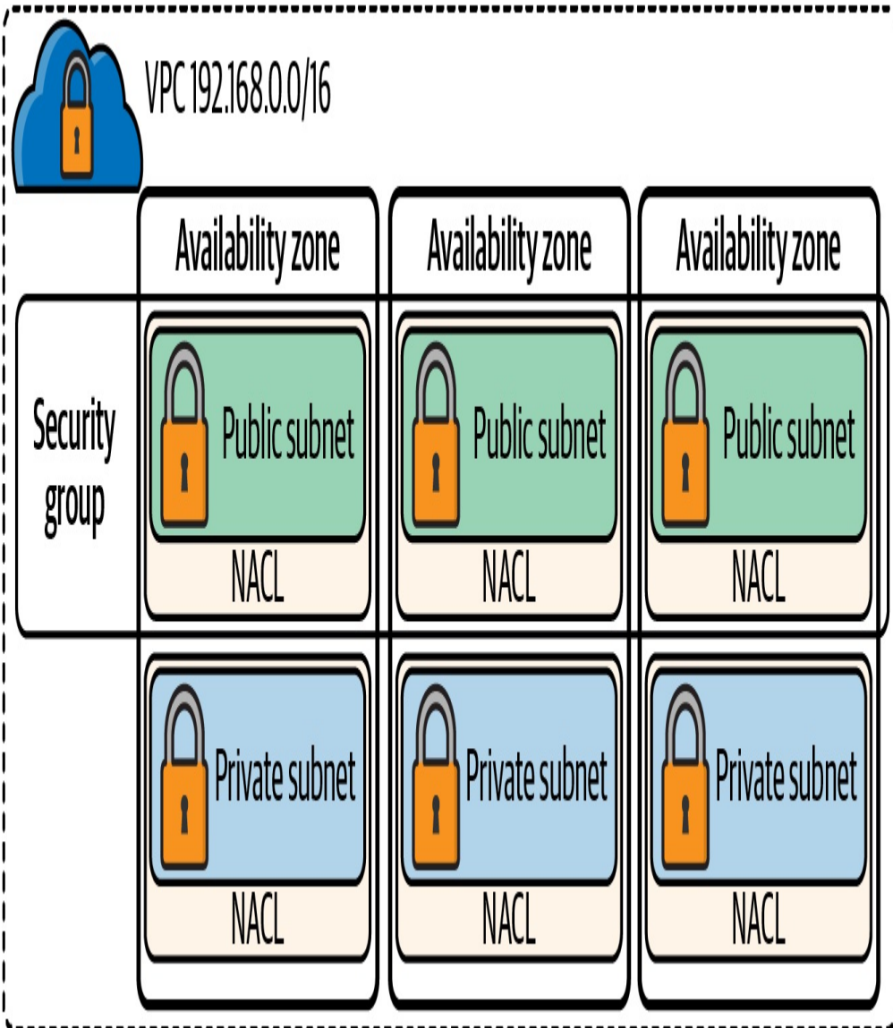
Figure 6-6. NACL
