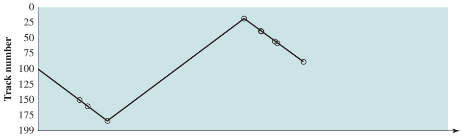
Time (d) C-SCAN
